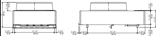
Zij aanzicht
